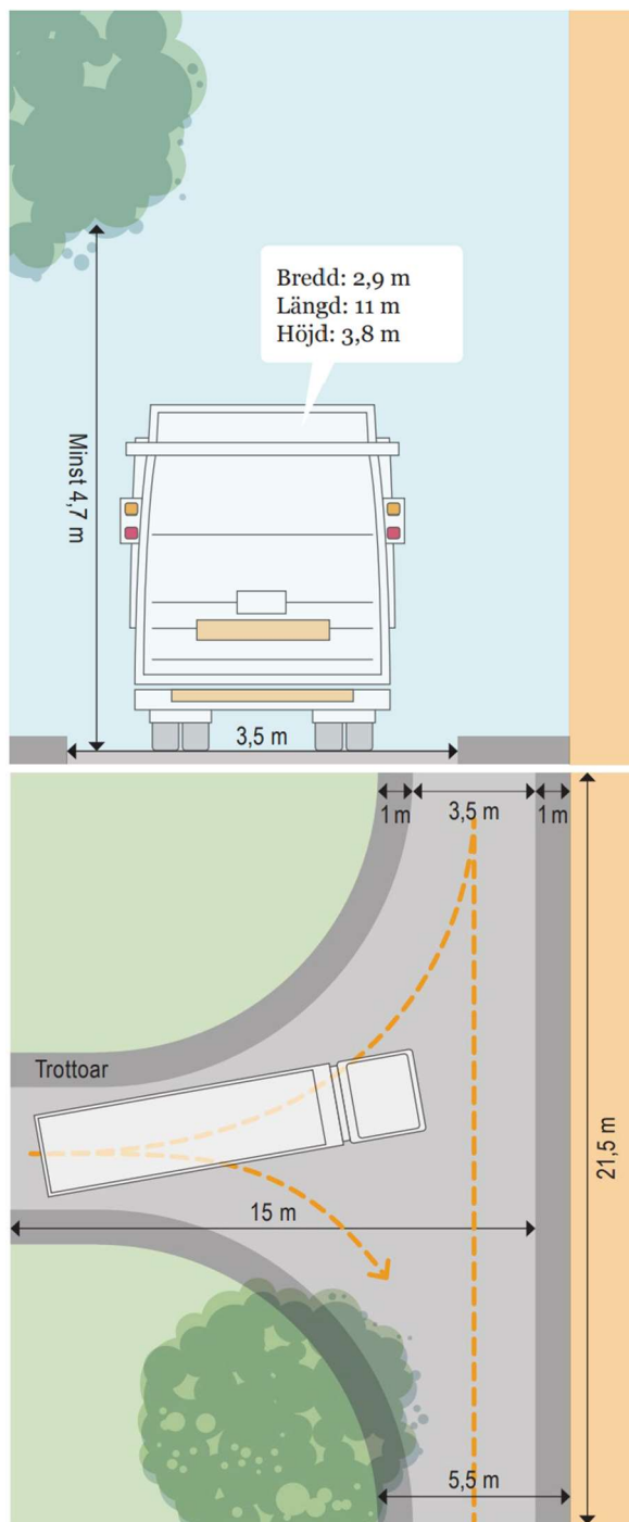
Figur 1. Transportvägens mått och vändplats i trevägskorsning (Avfall Sverige, 2018).
